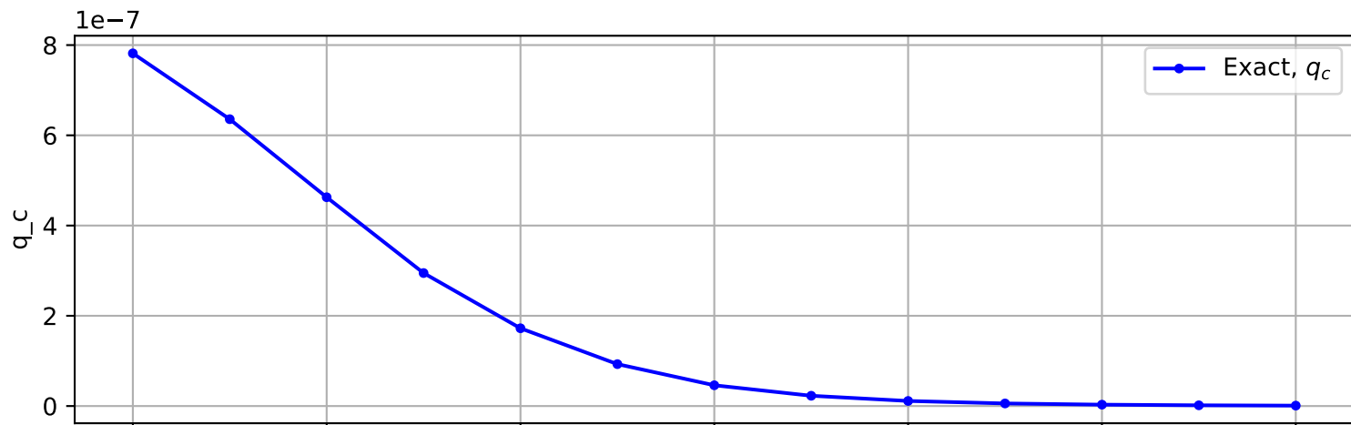
Trajectory No. 521
