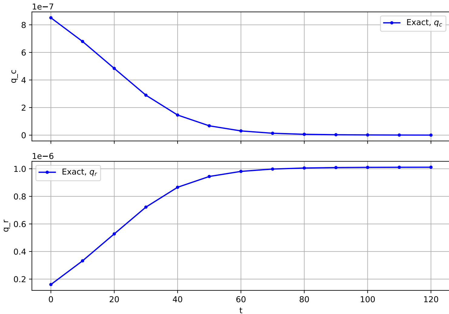
Trajectory No. 571
