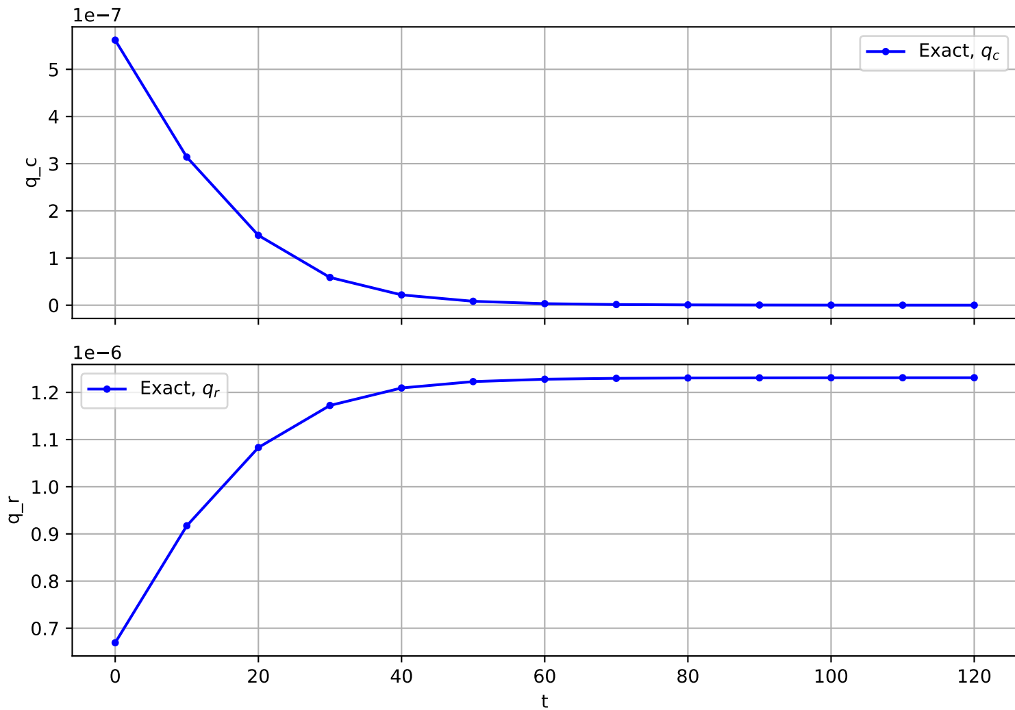
Trajectory No. 590
