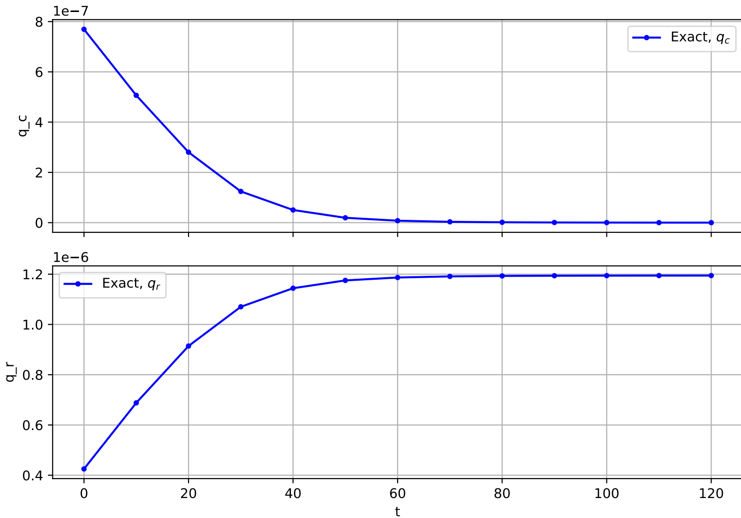
Trajectory No. 598
