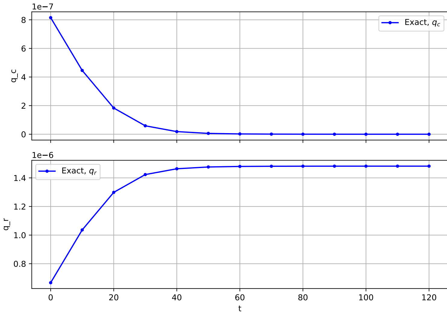
Trajectory No. 628
