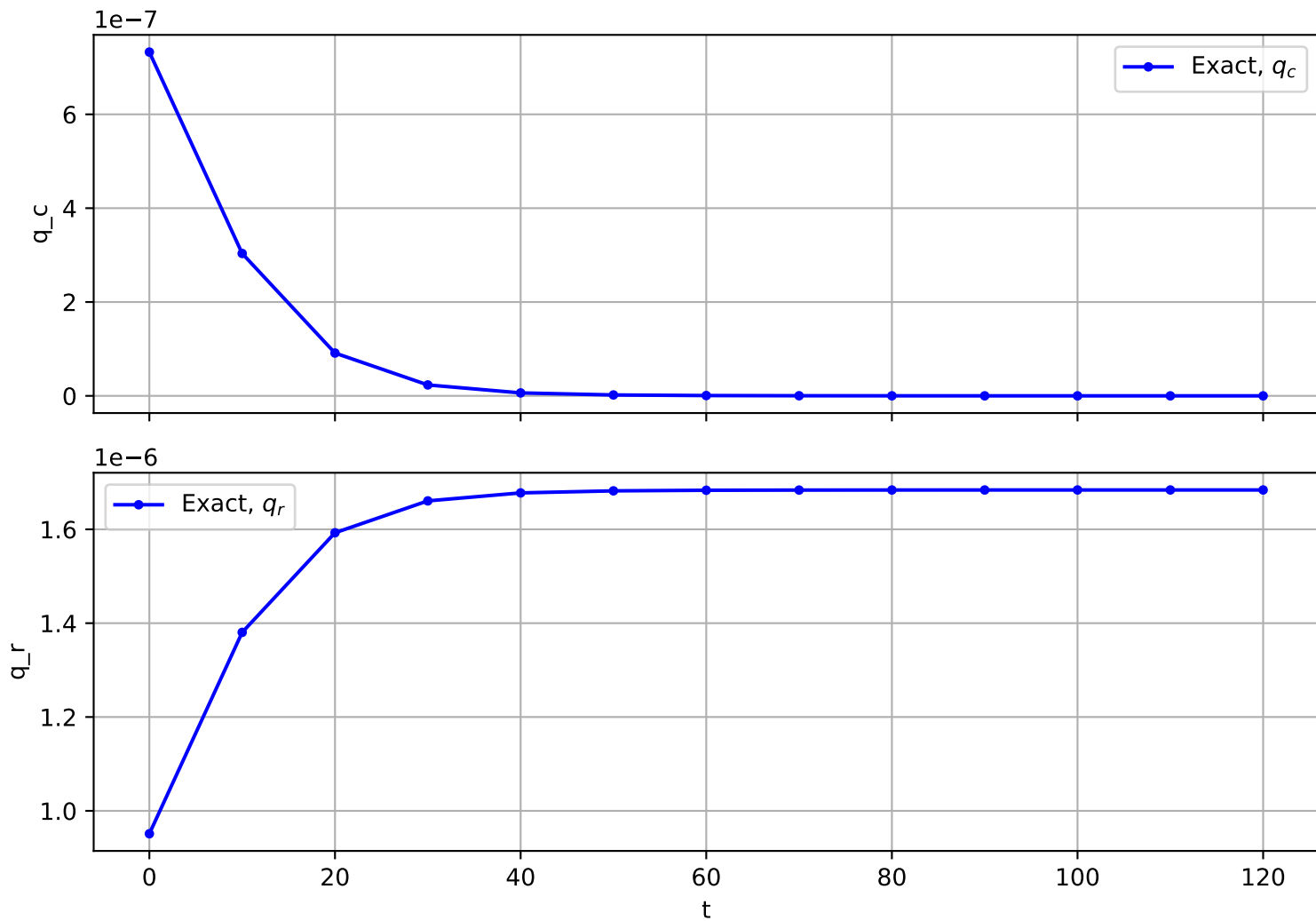
Trajectory No. 668
