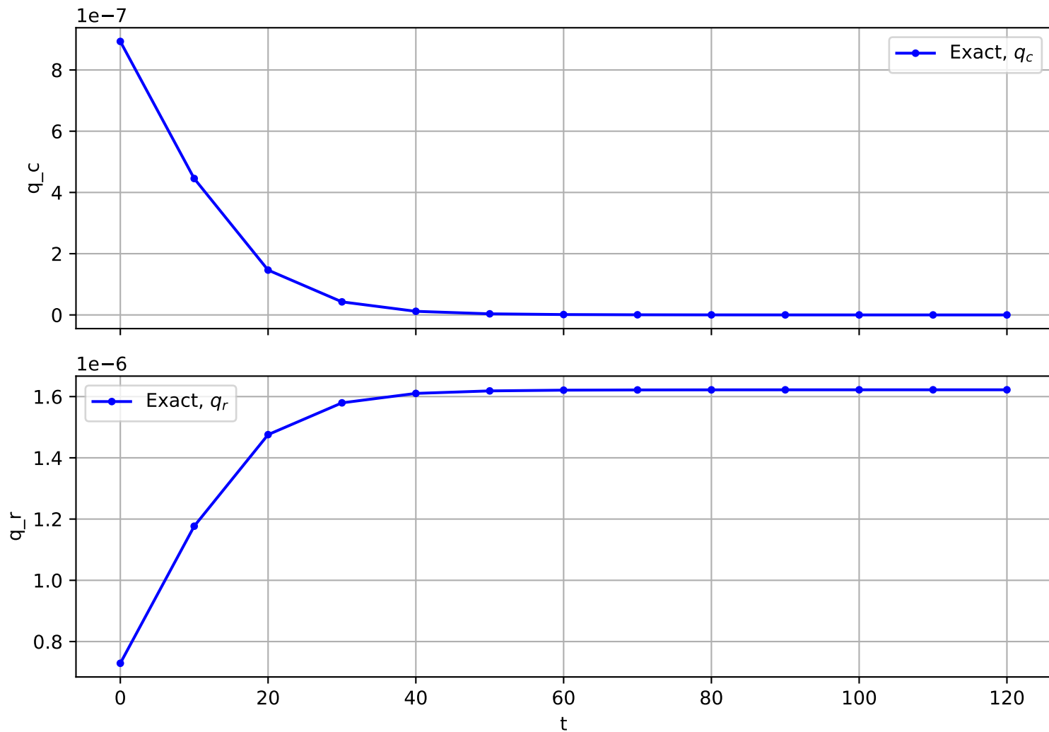
Trajectory No. 673
