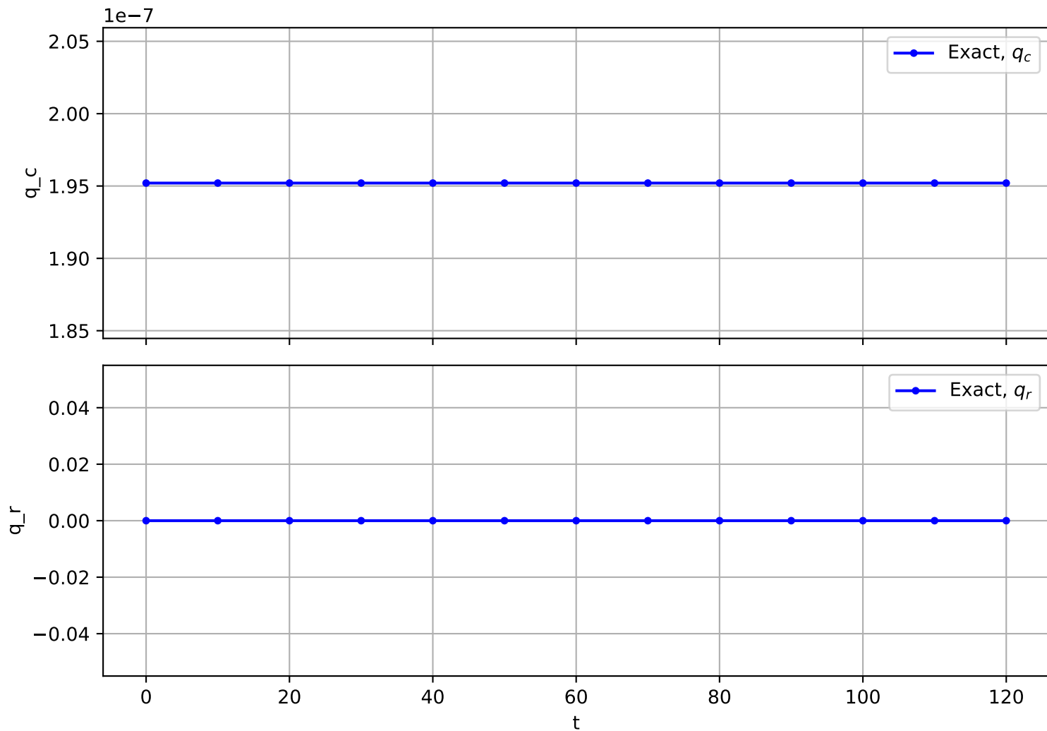
Trajectory No. 721
