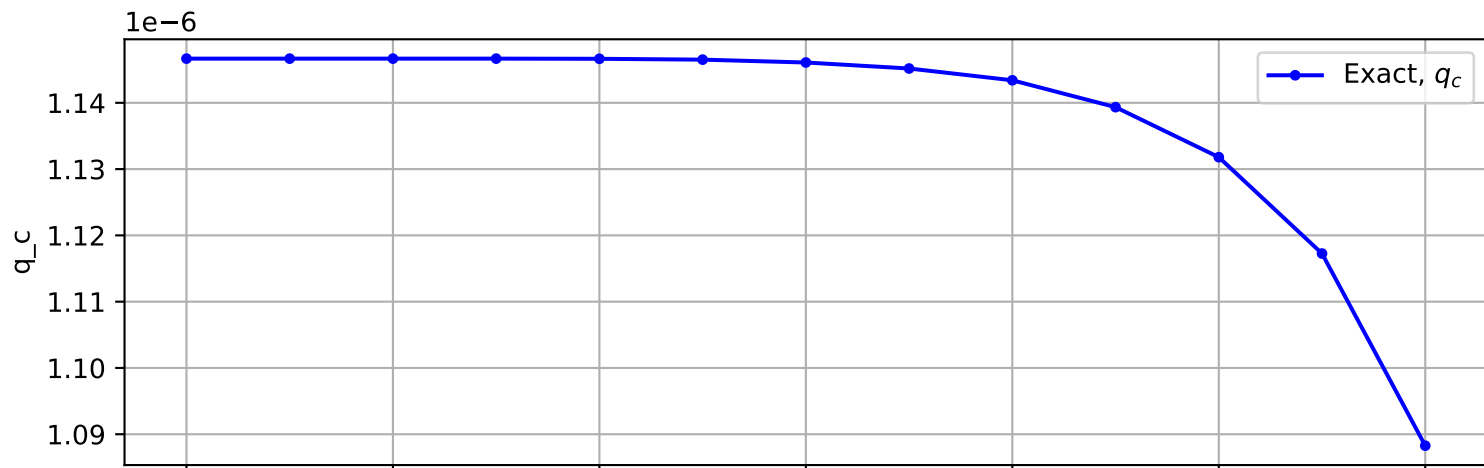
Trajectory No. 803
