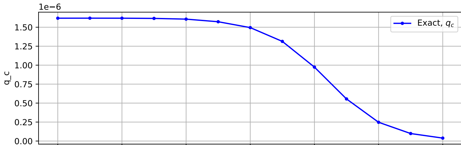
Trajectory No. 862
