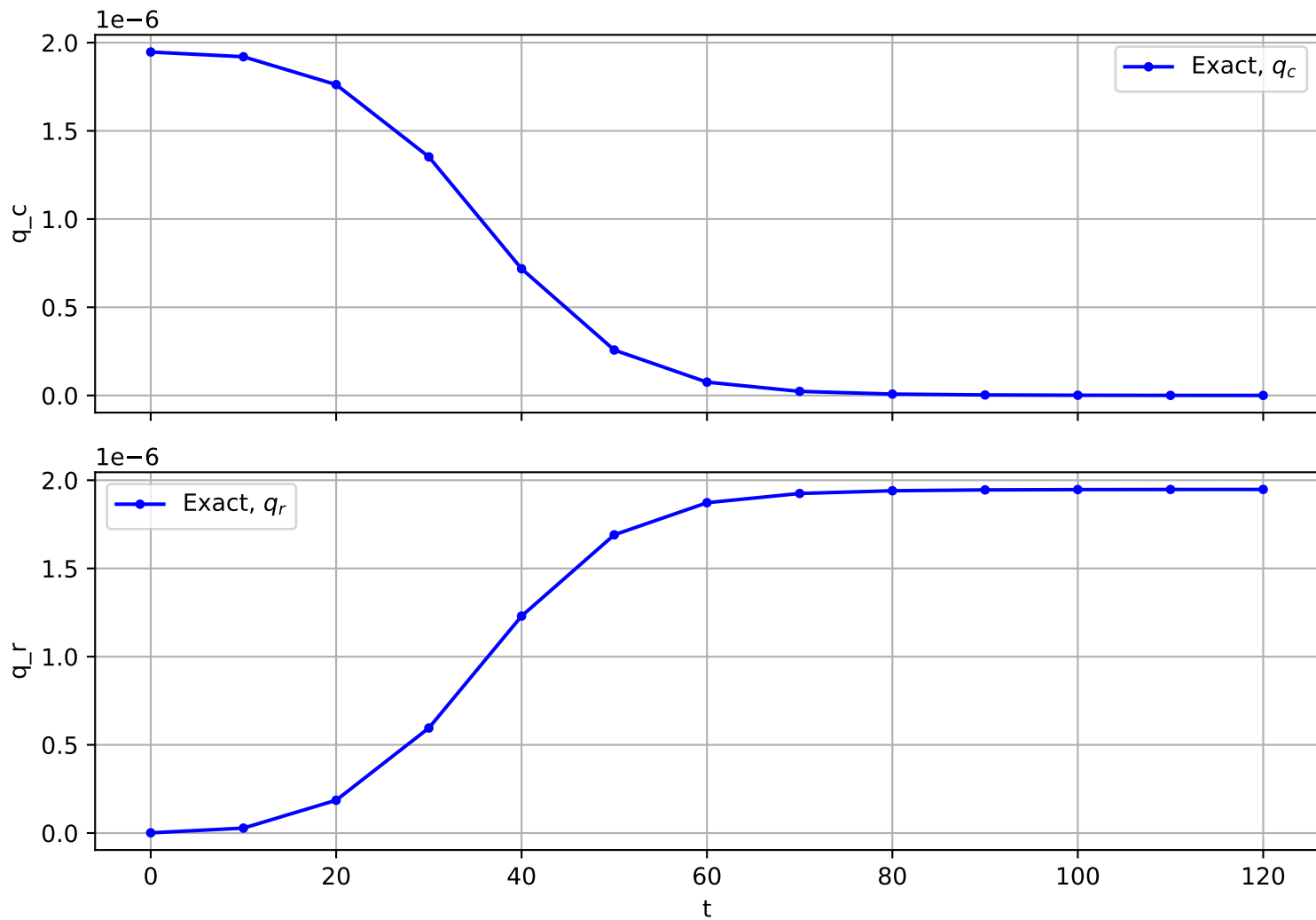
Trajectory No. 887
