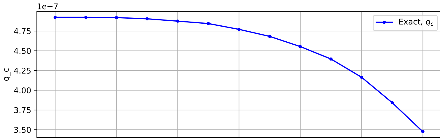
Trajectory No. 998
