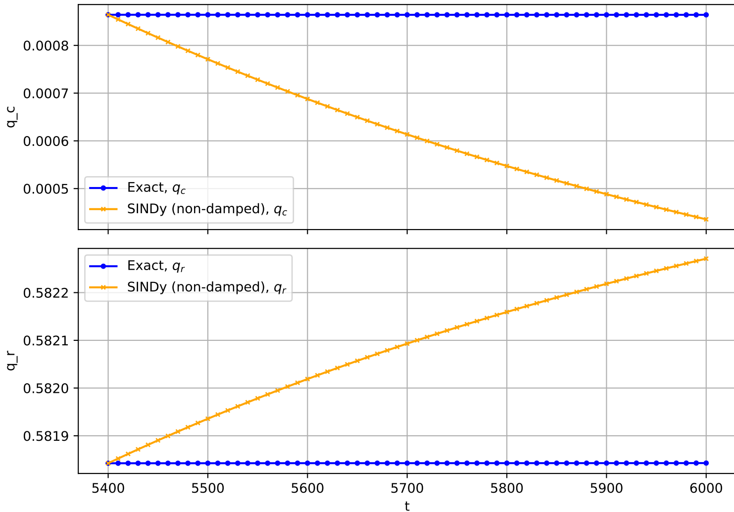
Trajectory No. 1006
