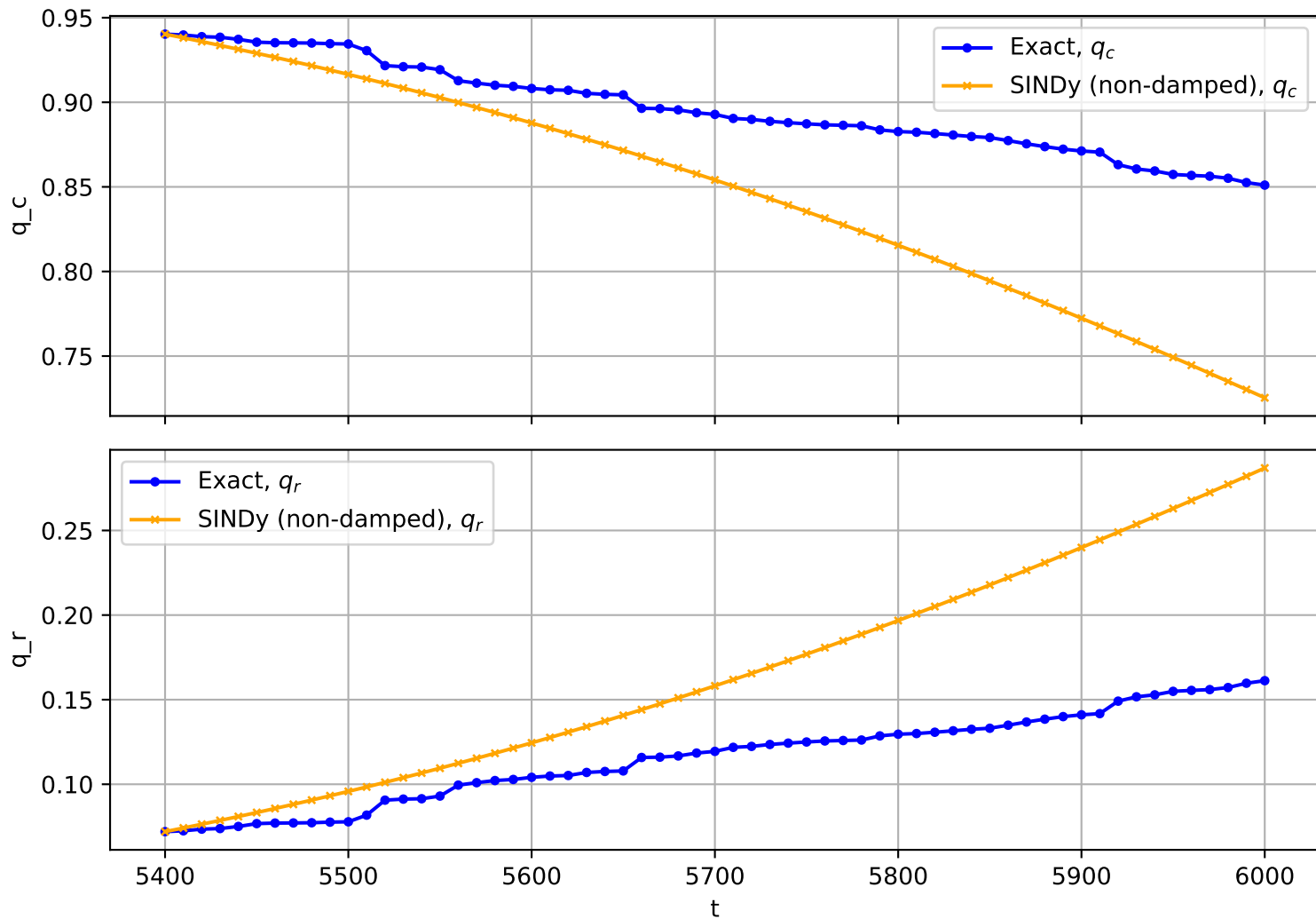
Trajectory No. 1009
