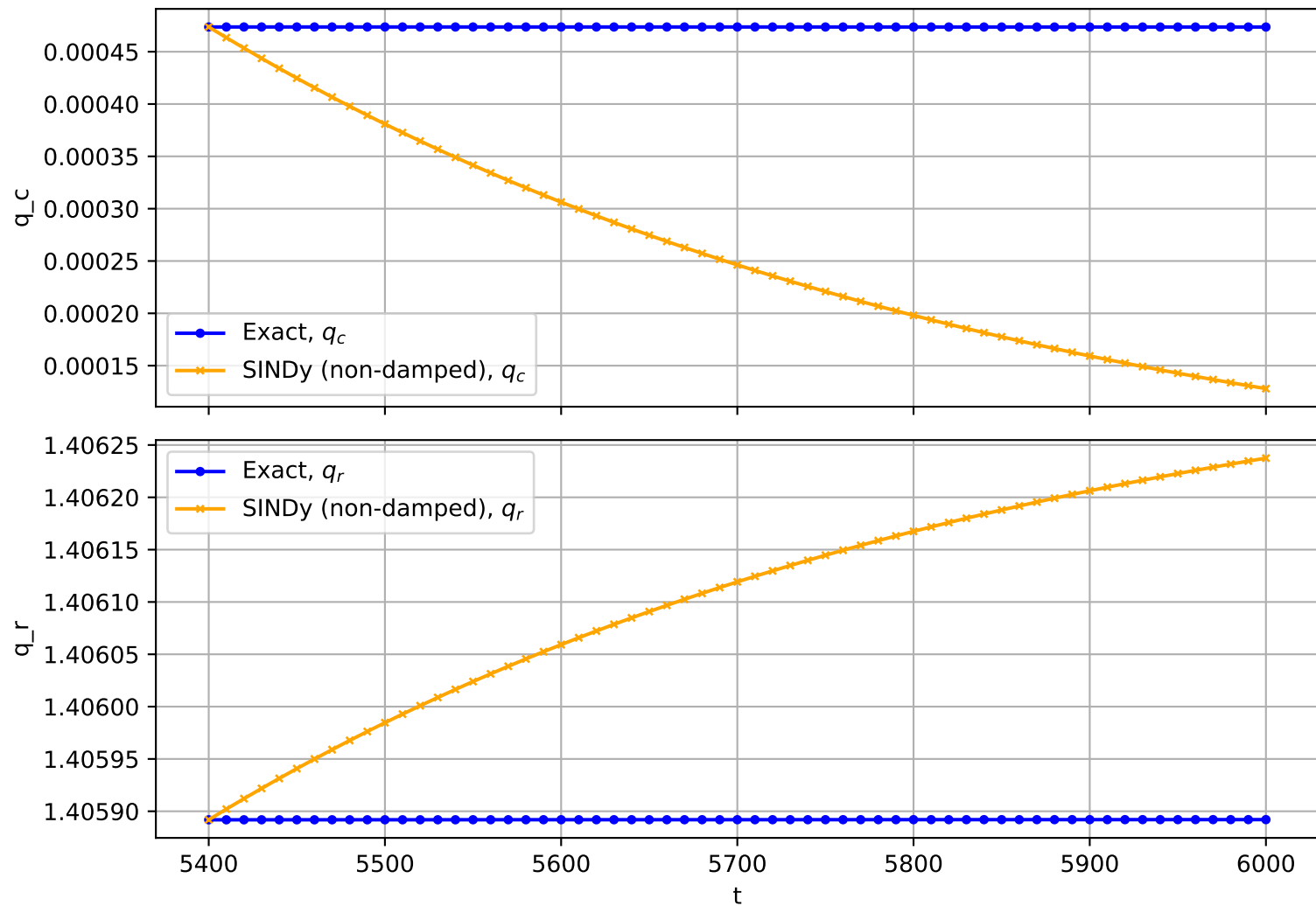
Trajectory No. 1069
