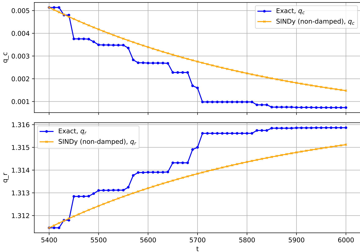
Trajectory No. 1074
