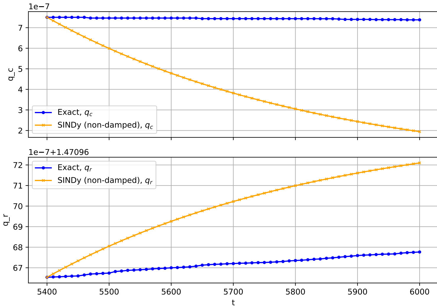
Trajectory No. 1092
