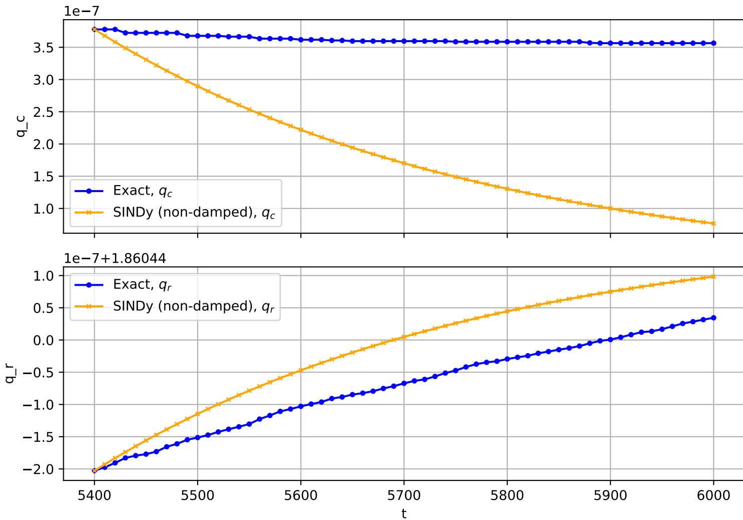
Trajectory No. 1114
