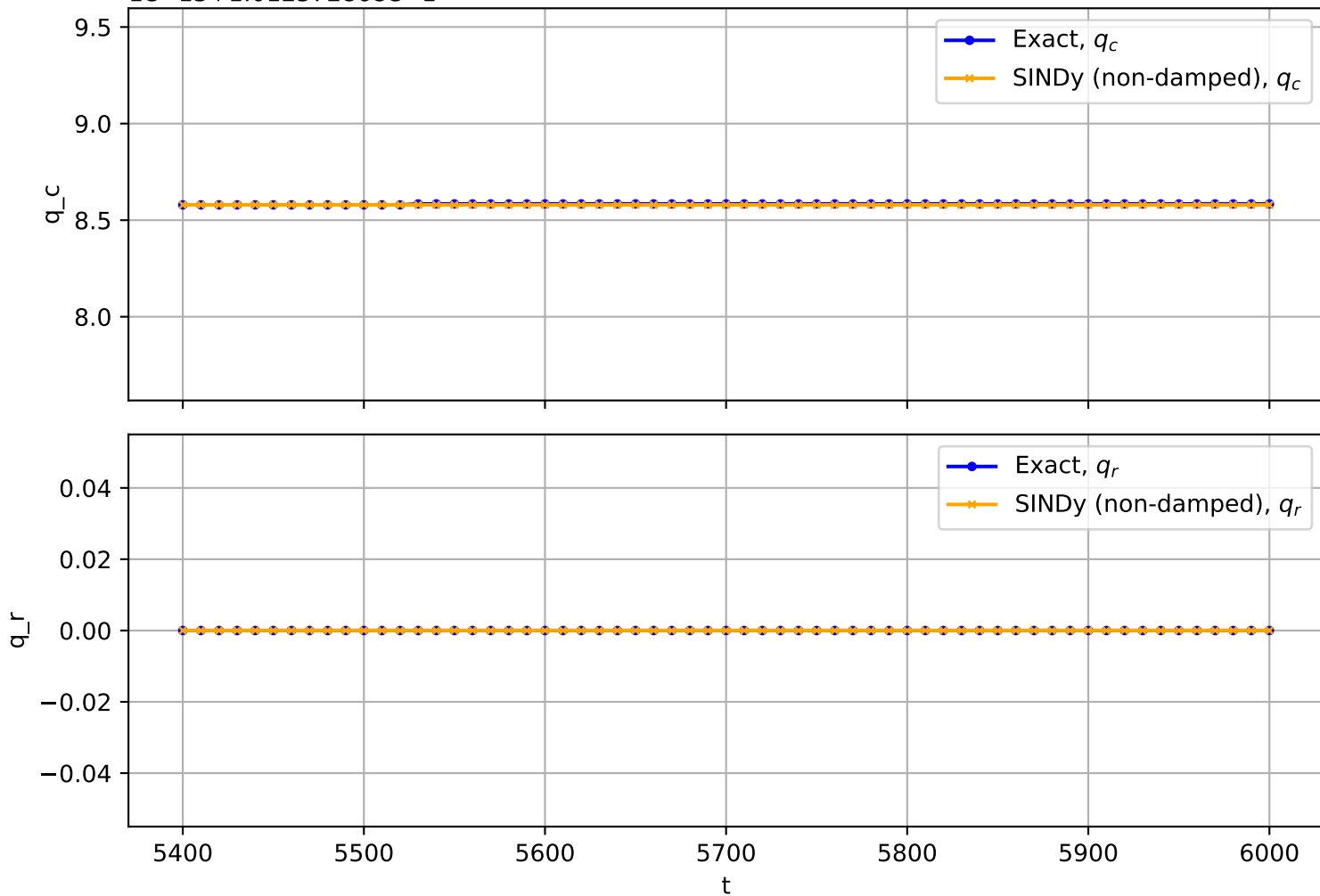
Trajectory No. 1129
