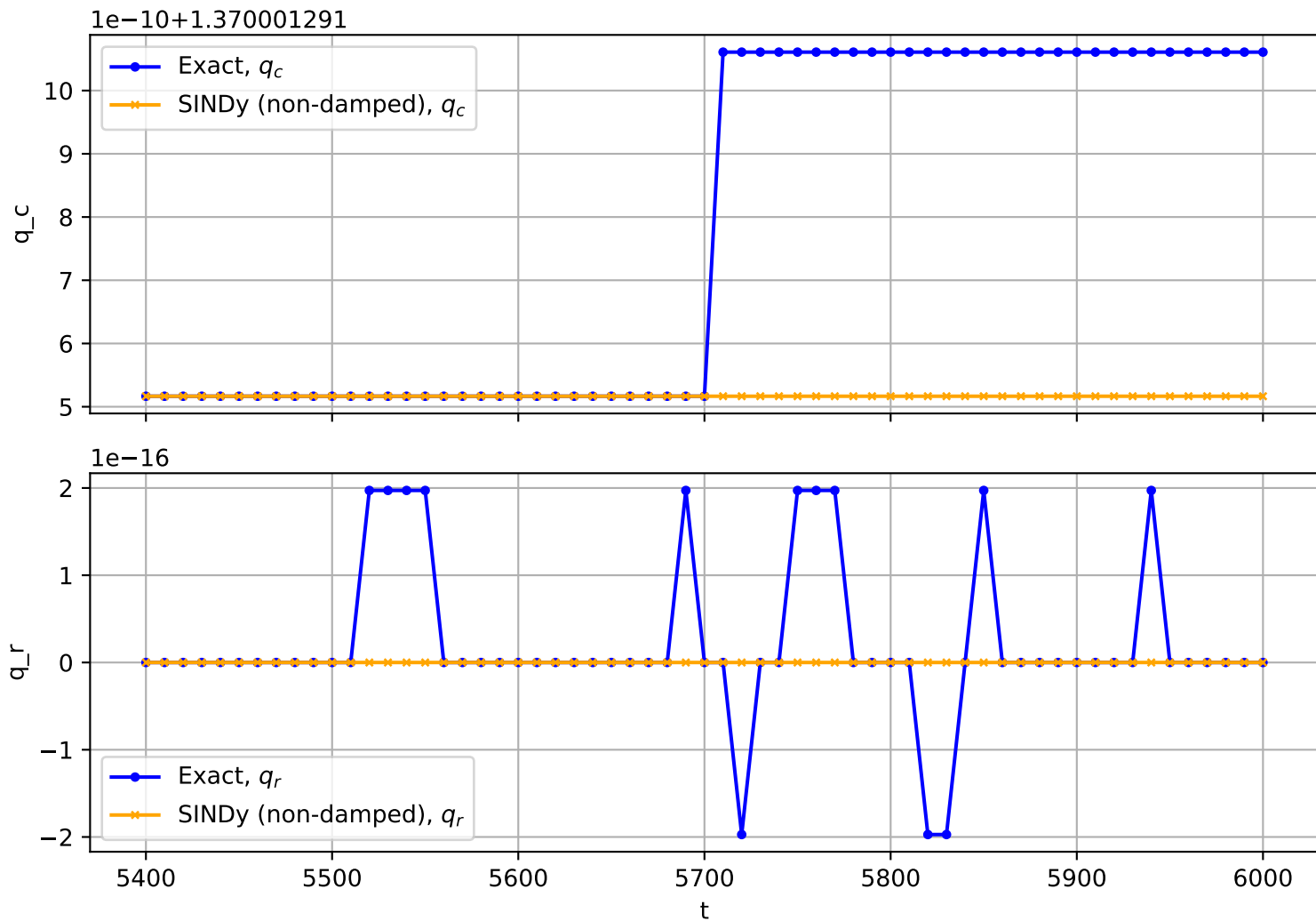
Trajectory No. 1138
