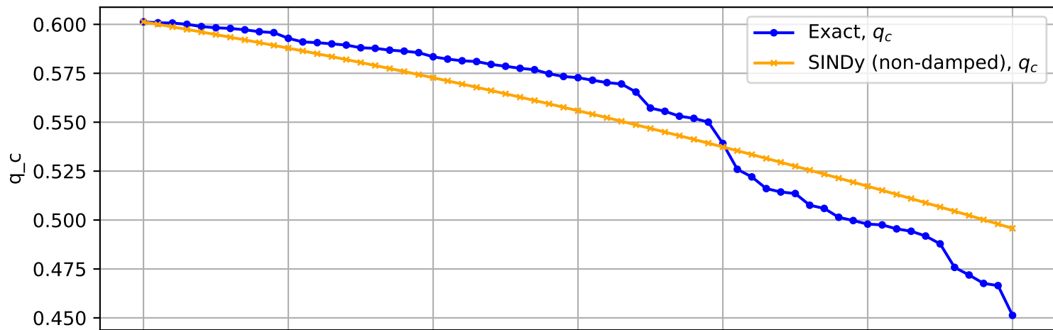
Trajectory No. 1154
