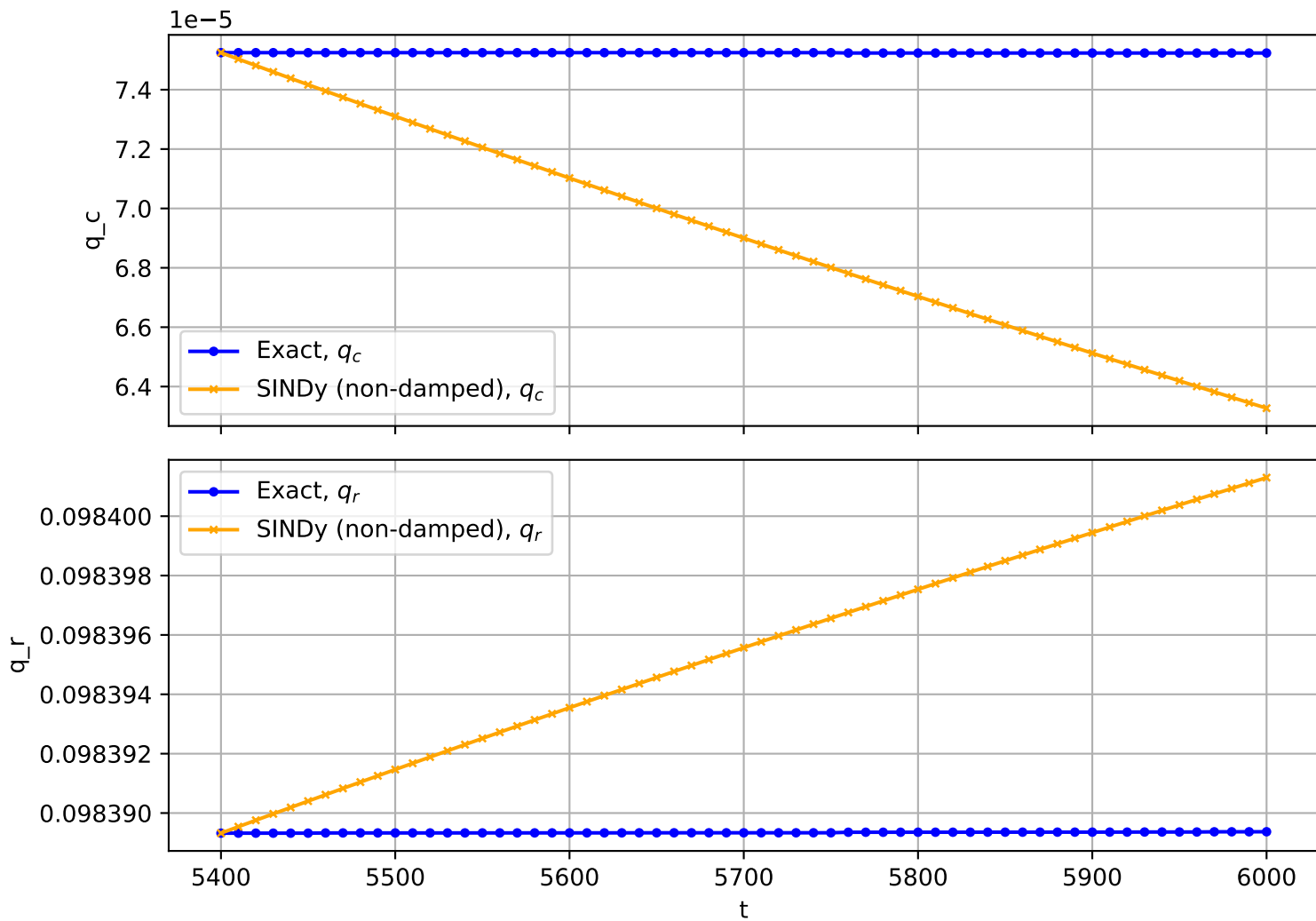
Trajectory No. 1272
