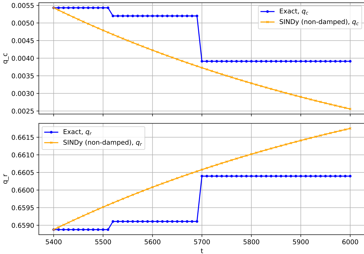
Trajectory No. 1396
