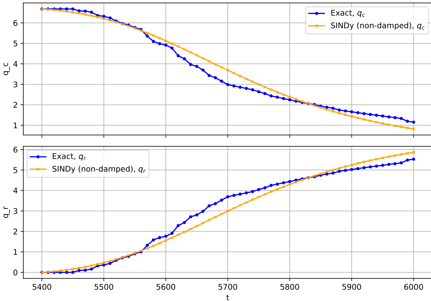
Trajectory No. 1419
