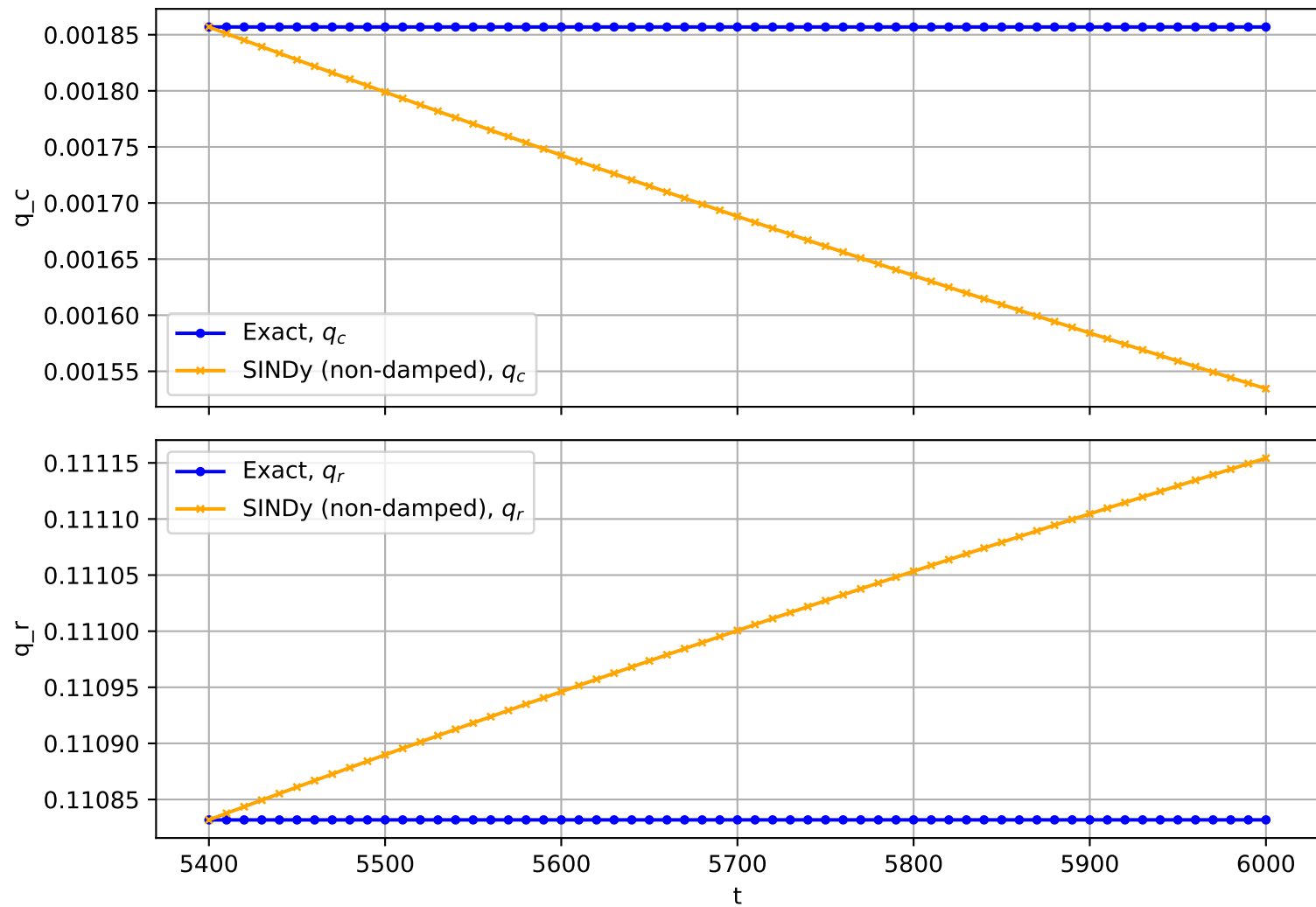
Trajectory No. 1436
