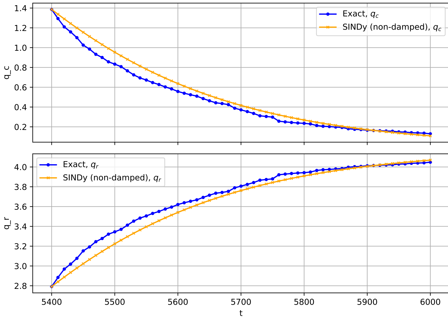
Trajectory No. 1469
