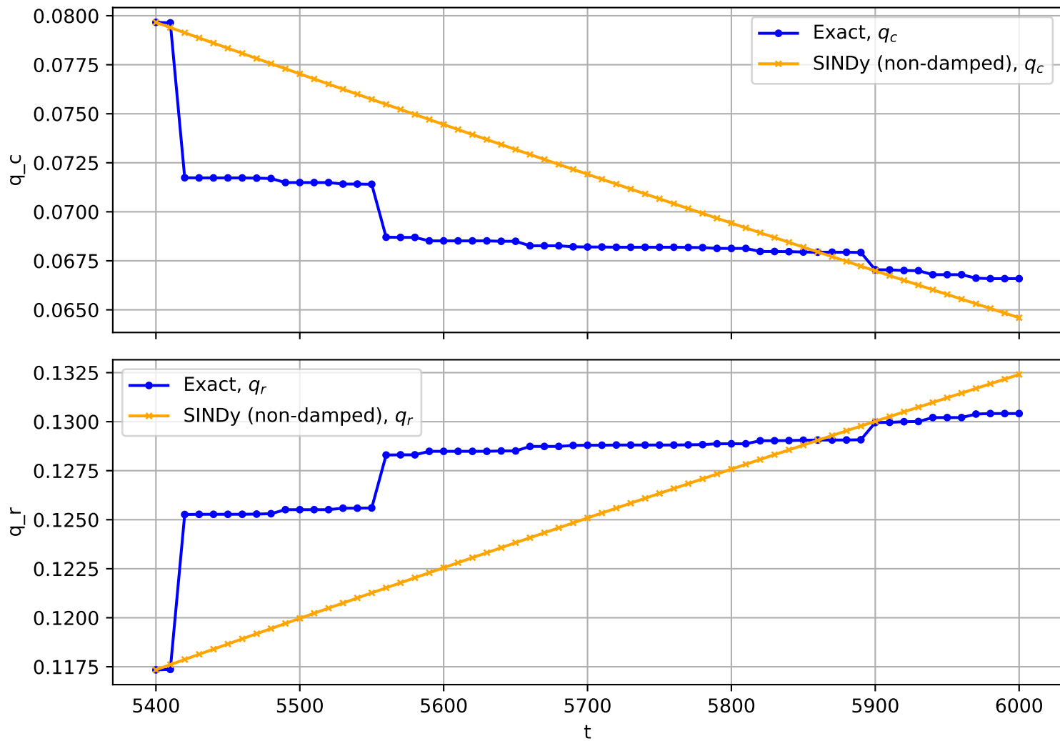
Trajectory No. 1472
