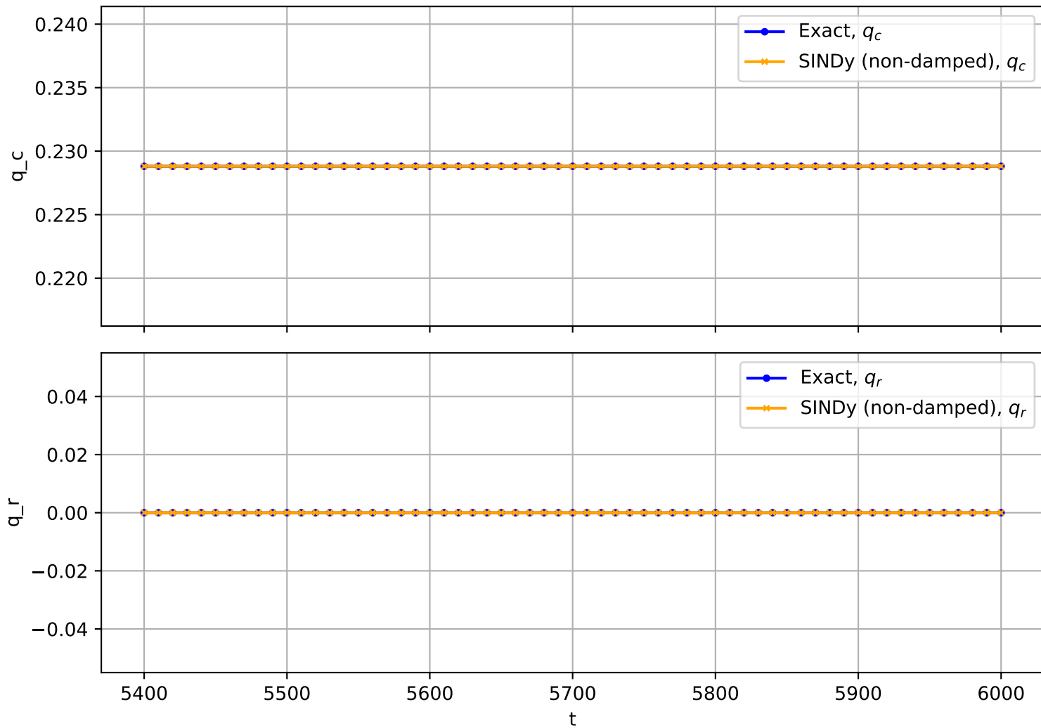
Trajectory No. 1541
