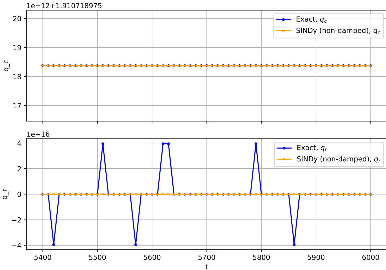
Trajectory No. 1608
