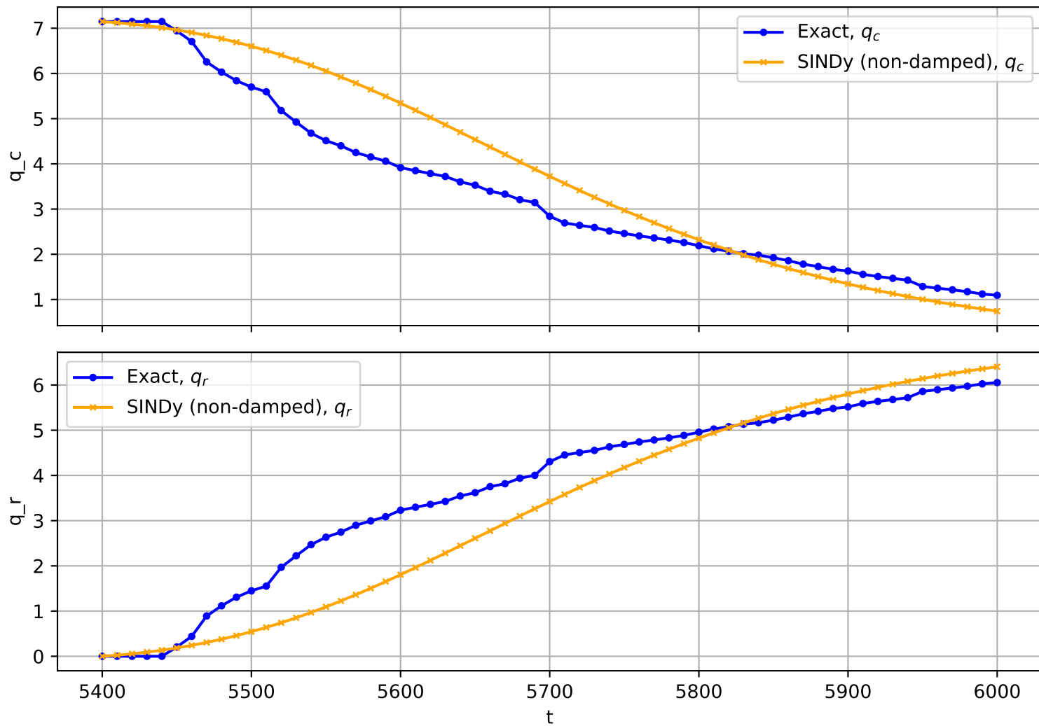
Trajectory No. 1649
