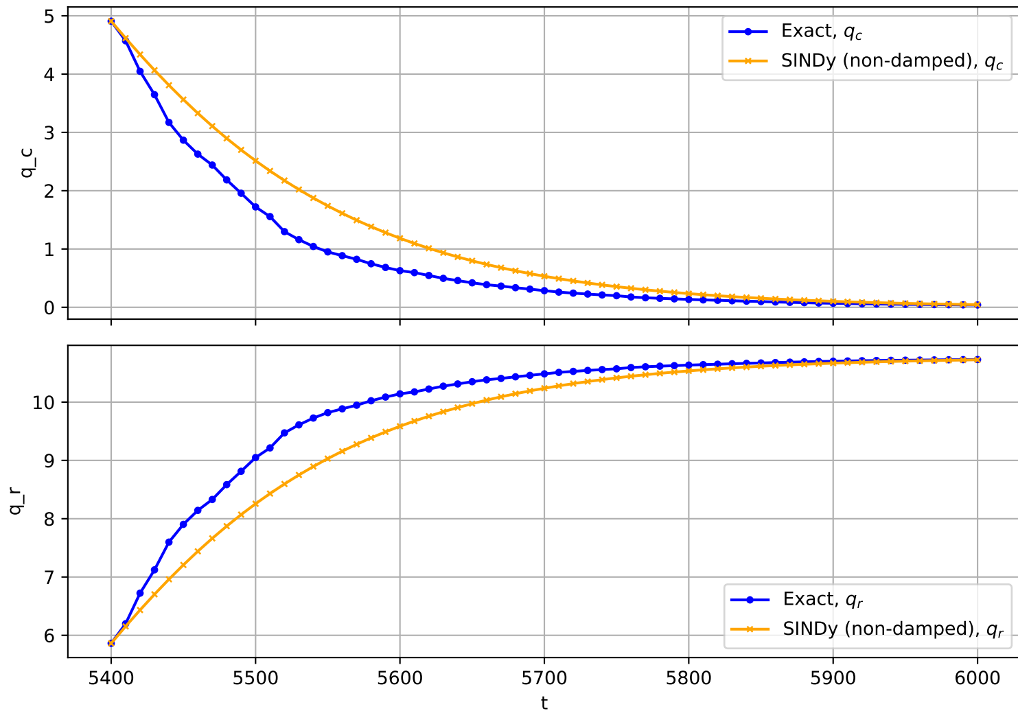
Trajectory No. 1698
