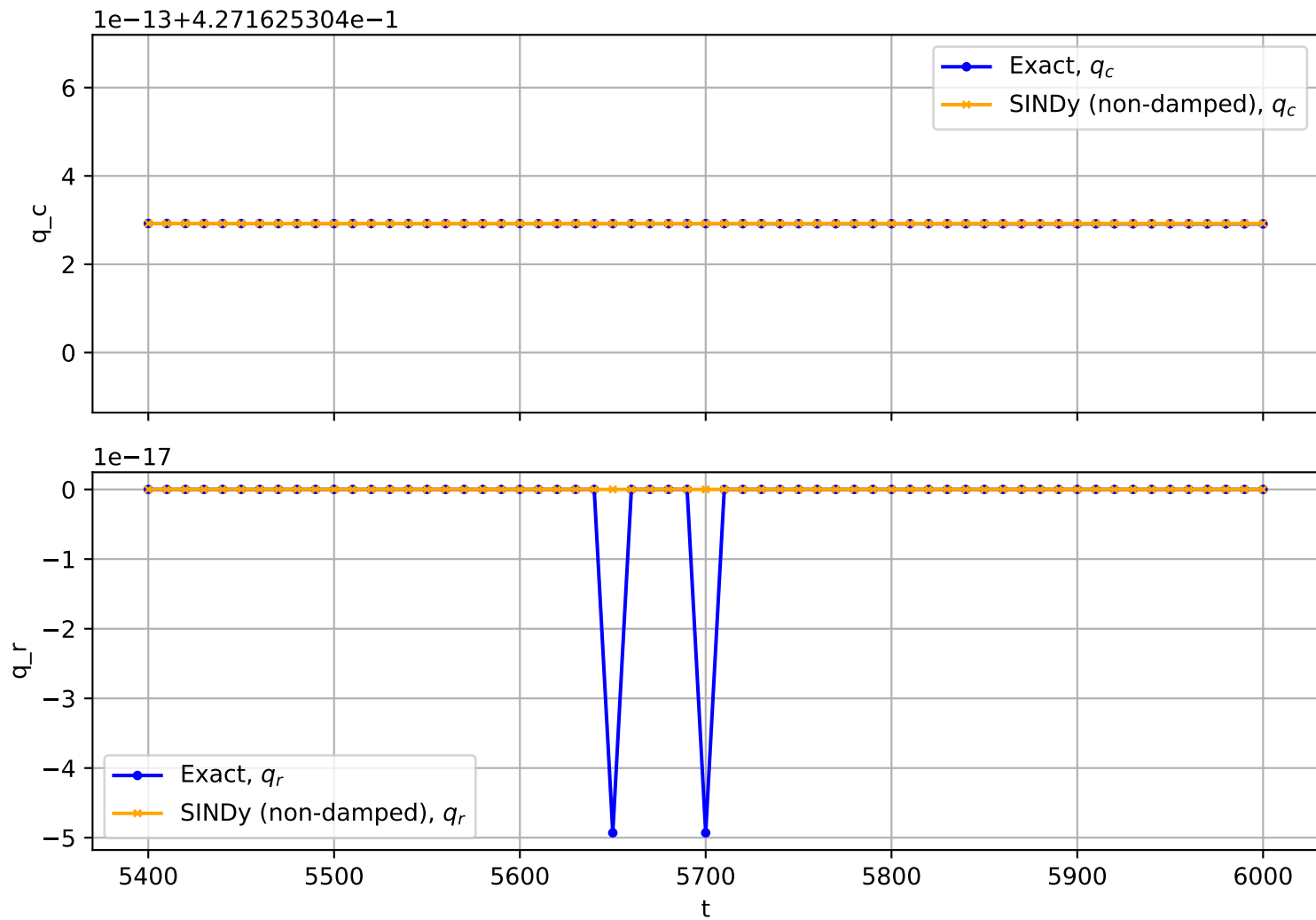
Trajectory No. 1760
