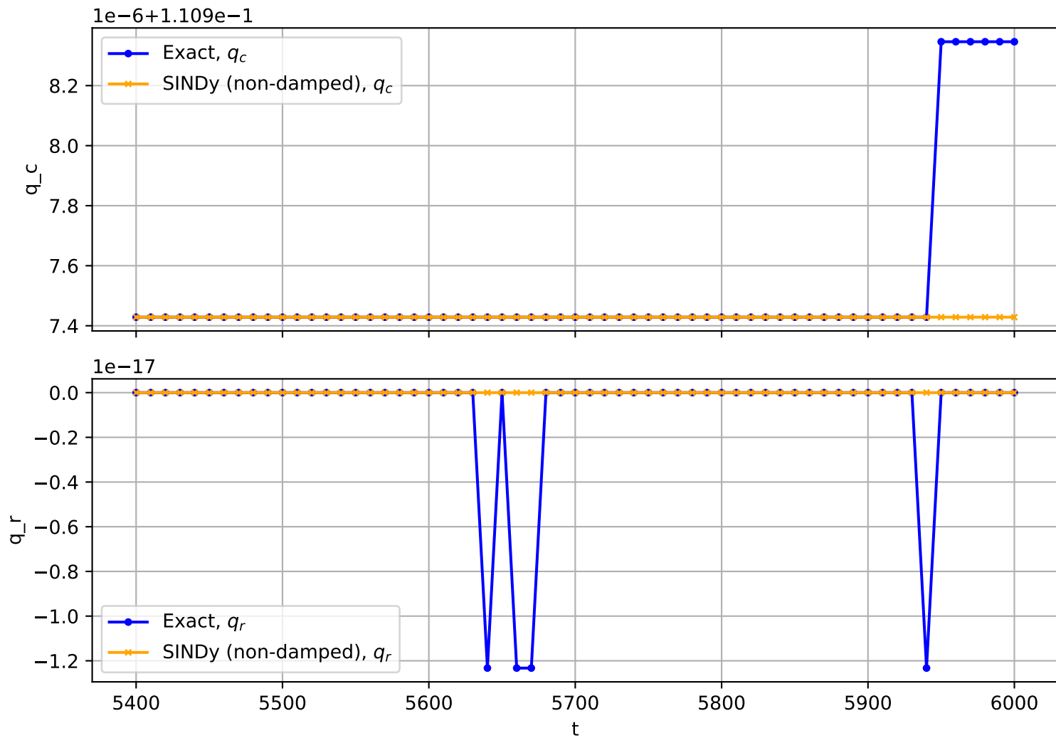
Trajectory No. 1784
