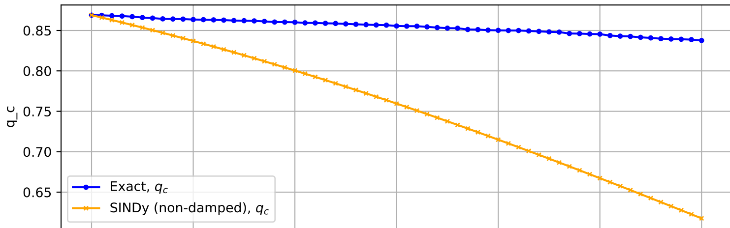
Trajectory No. 189
