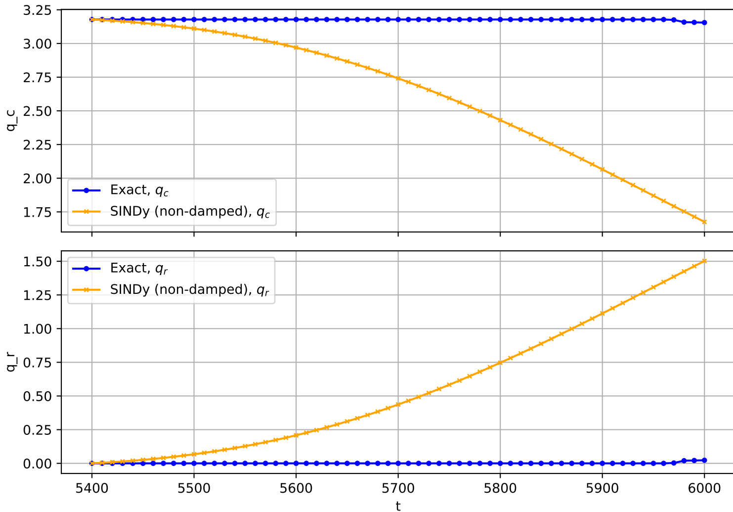
Trajectory No. 2036
