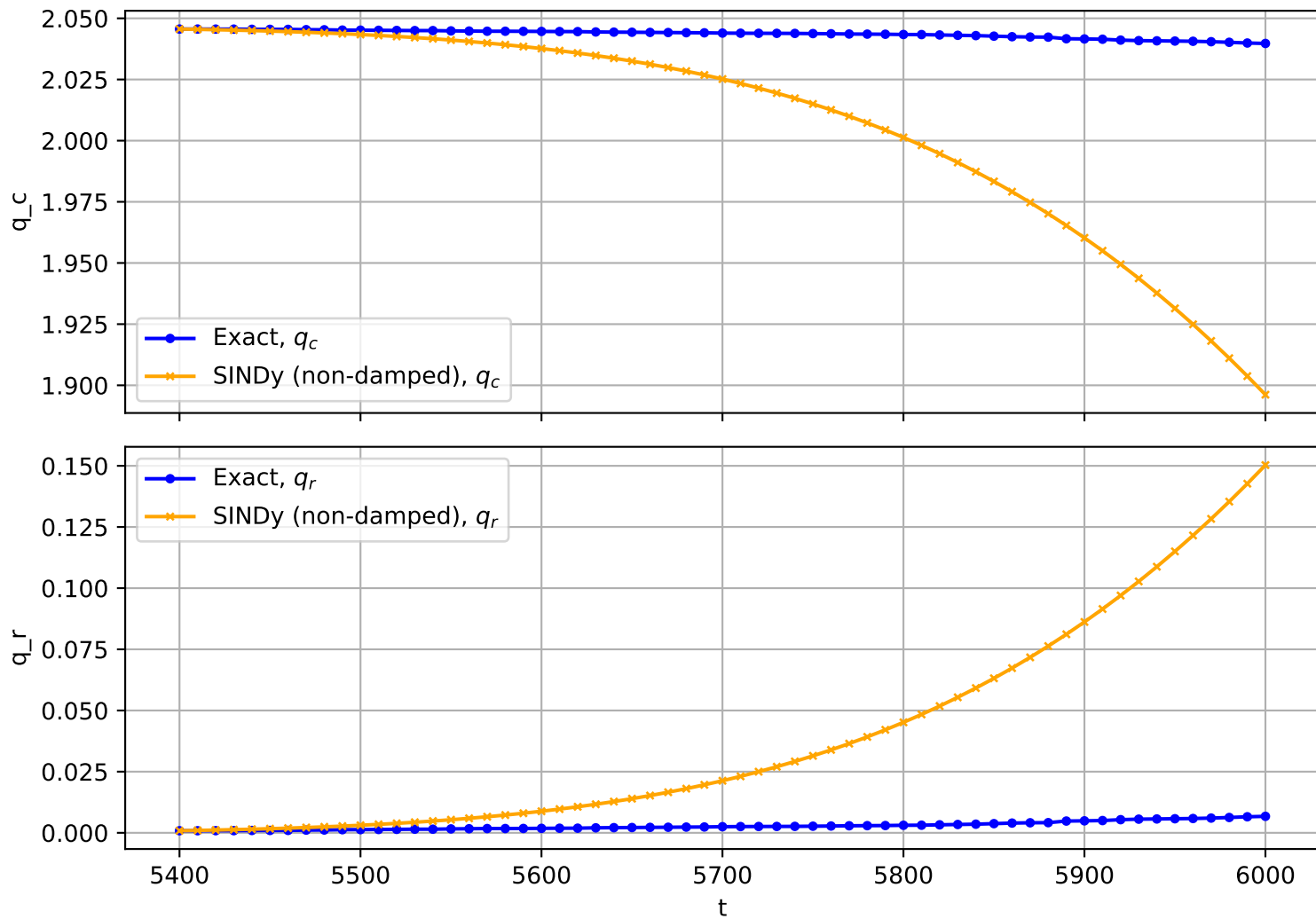
Trajectory No. 2052
