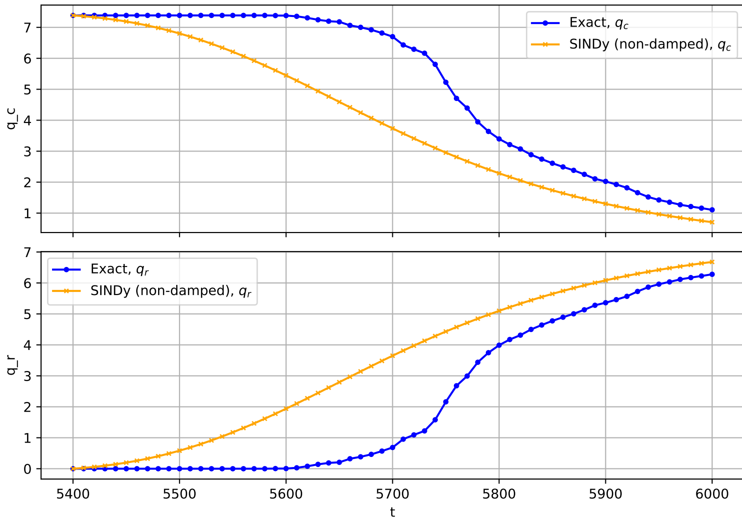
Trajectory No. 2096
