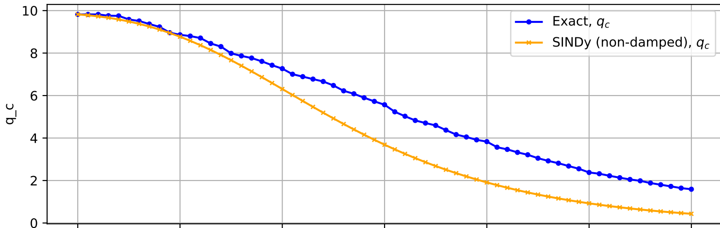
Trajectory No. 2150
