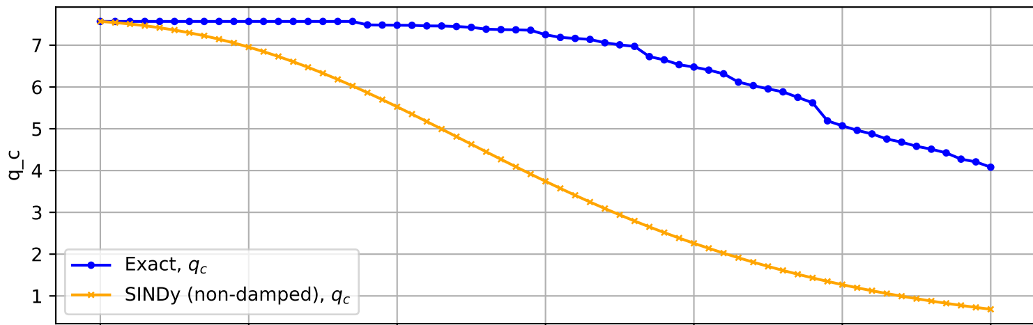
Trajectory No. 2157
