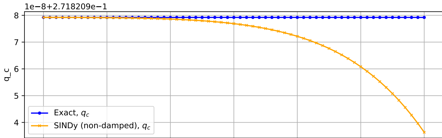
Trajectory No. 2198
