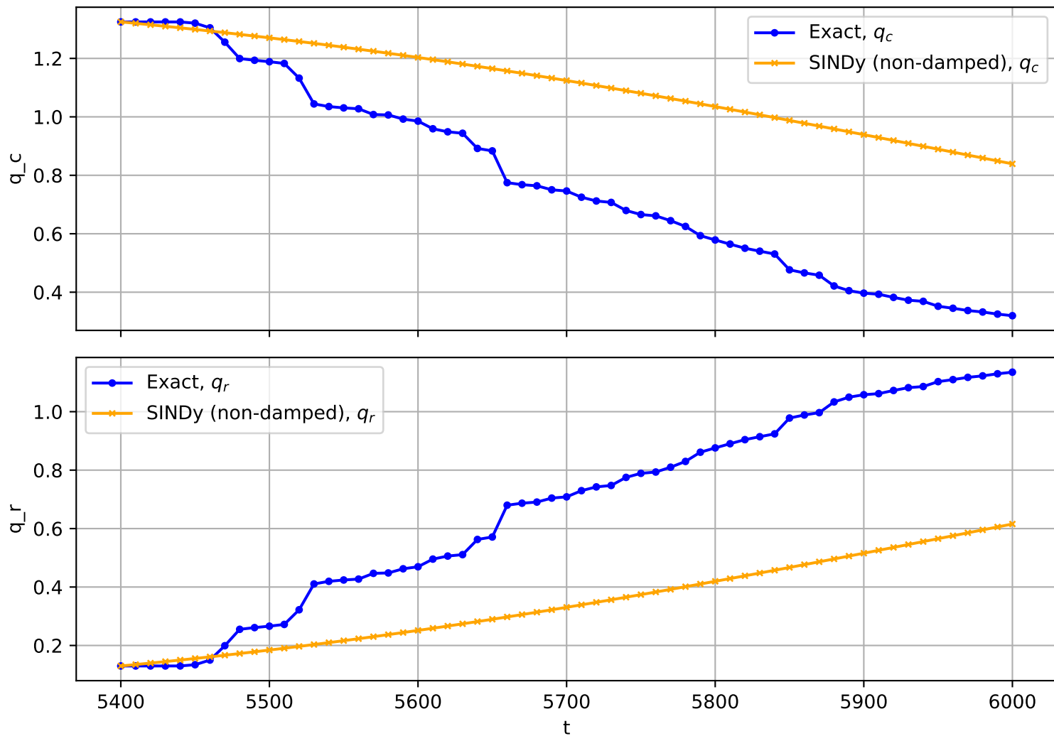
Trajectory No. 2217
