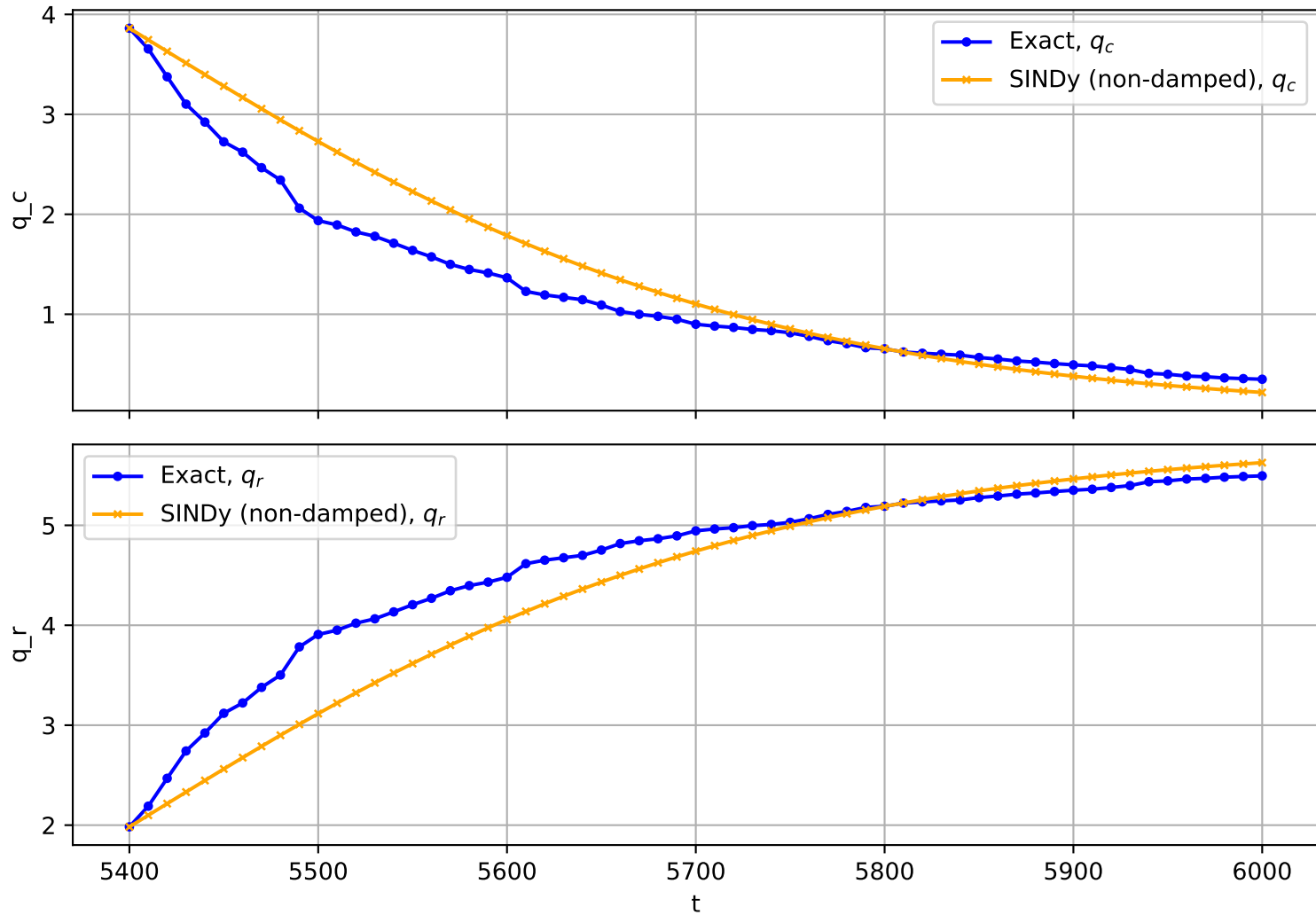
Trajectory No. 2219
