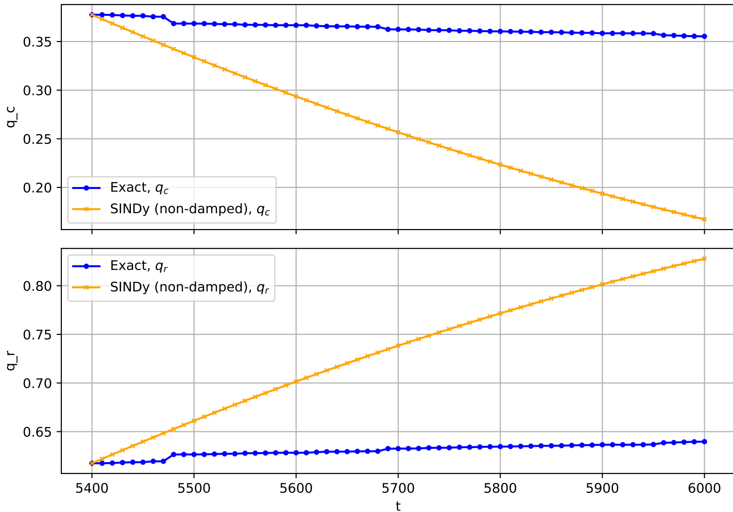
Trajectory No. 2222
