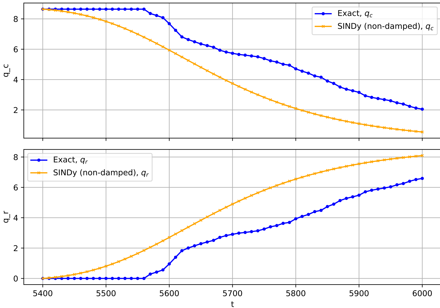
Trajectory No. 2245
