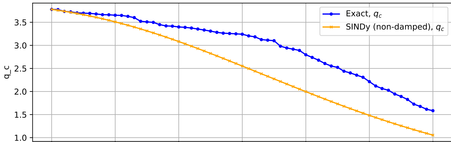
Trajectory No. 2267
