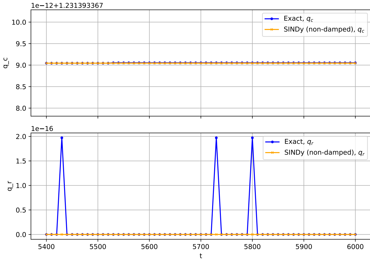
Trajectory No. 227
