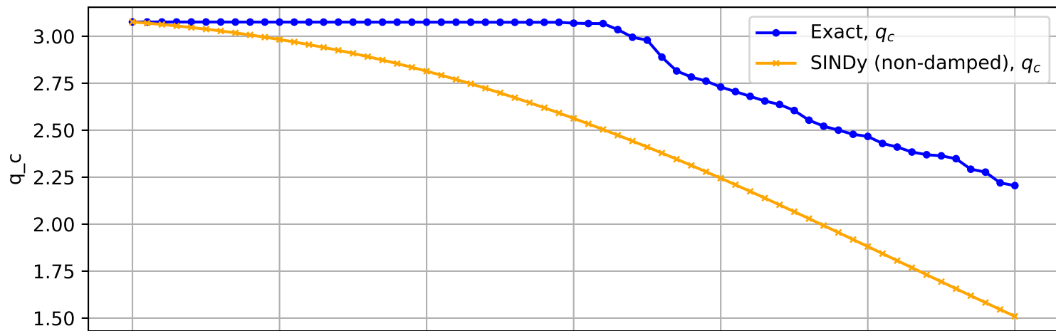
Trajectory No. 2322
