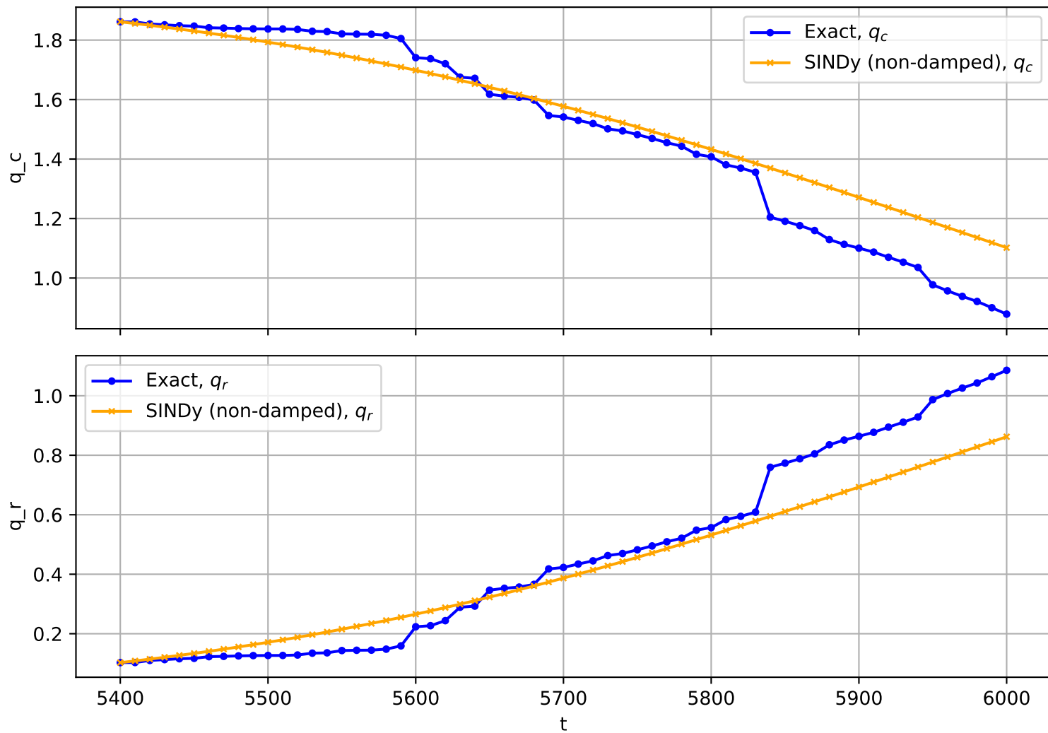
Trajectory No. 2371
