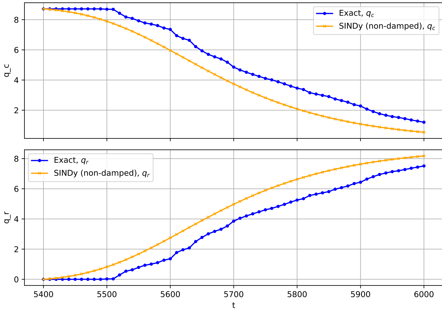
Trajectory No. 2374
