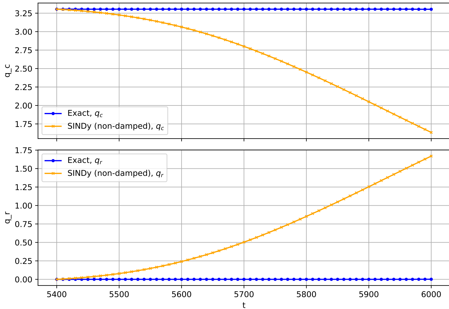
Trajectory No. 2408
